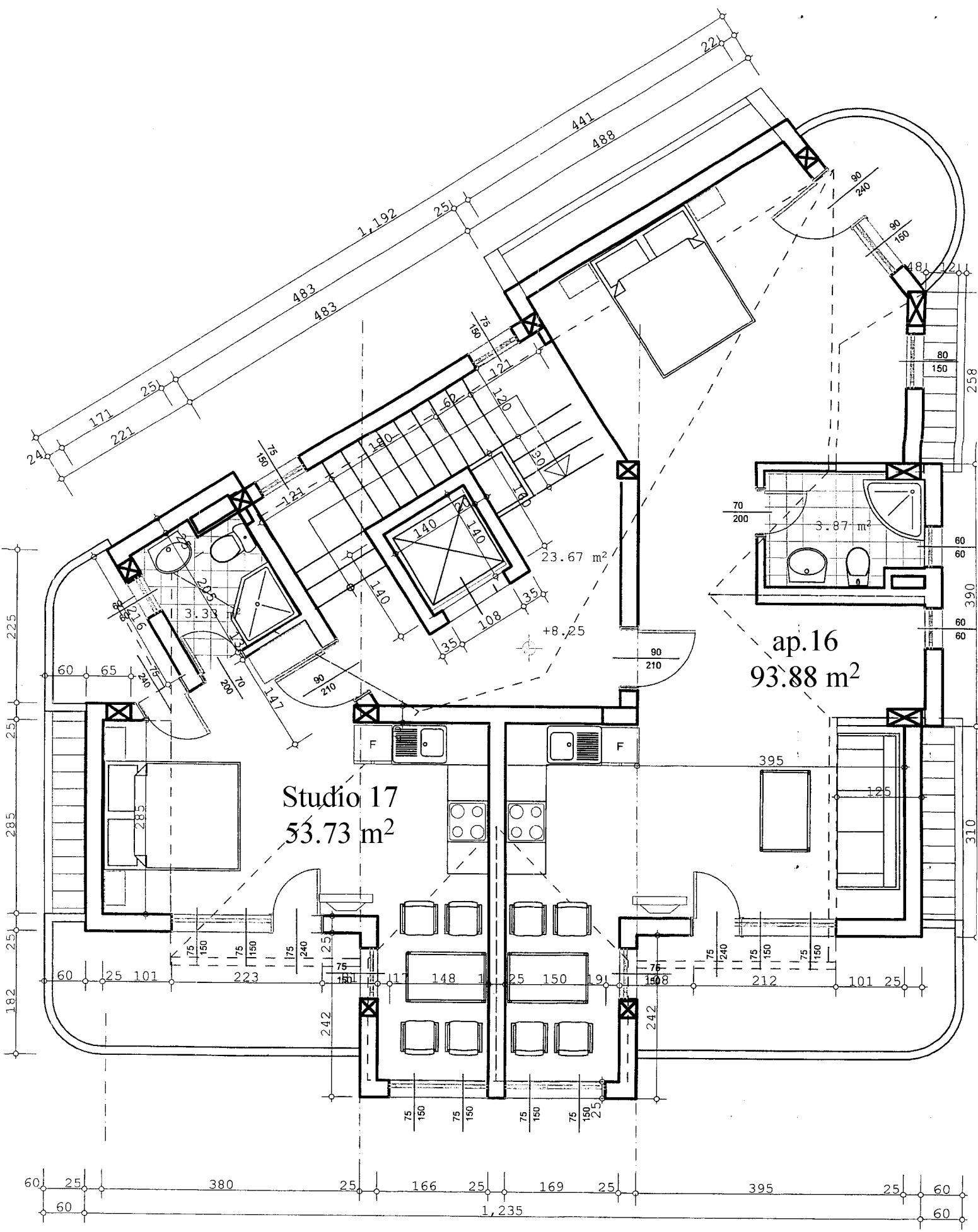
РАЗПРЕДЕЛЕНИЕ КОТА +8,25
